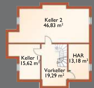
Kellergeschoss. Raumgröße gesamt 94,92 m 2
