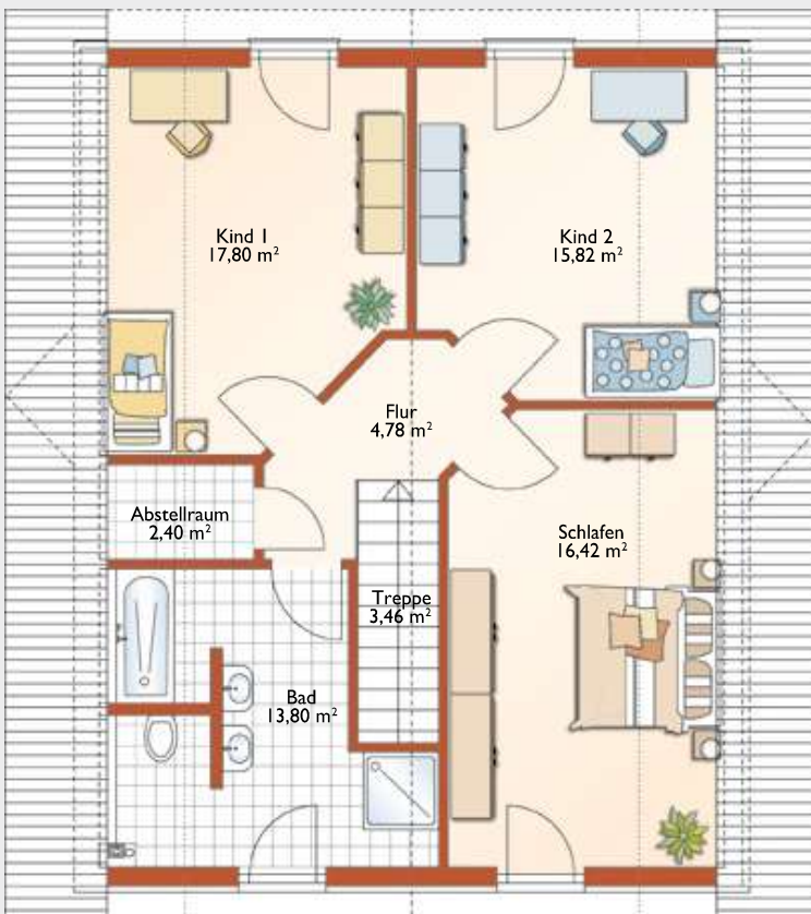
Dachgeschoss. Raumgröße gesamt 71,02 m 2
